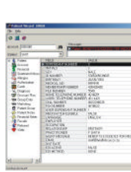
PatientRecords
